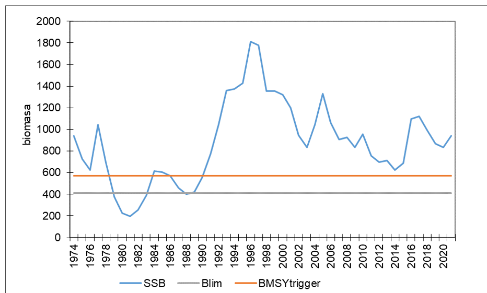
Rysunek 3. Szprot 22-32. Biomasa stada tarłowego (tys. ton) wraz z naniesionymi wartościami referencyjnymi BMSYtrigger i Blim (wartość BMSYtrigger przyjęta jako Bpa) wg danych ICES (2022a,b)
