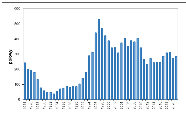
Rysunek 2. Szprot 22-32. Połowy (tys. ton) w okresie 1974-2021 wg danych ICES (2022a,b)
