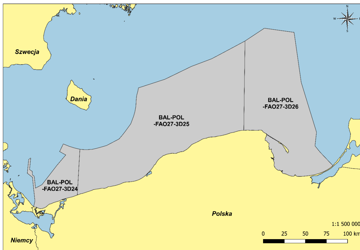
Rysunek 4. Obszary oceny w ramach wskaźnika ‘Biomasa stada tartłowego(szprot)’
