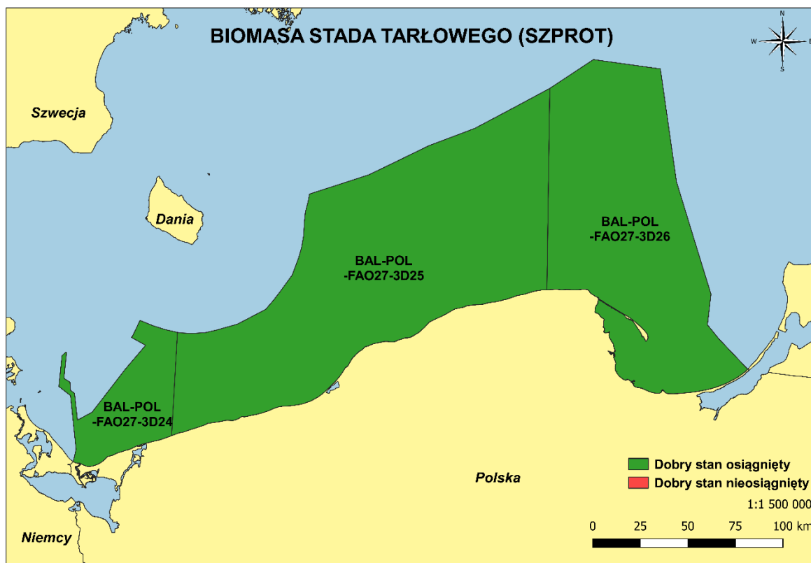
Rysunek 1. Ocena stanu środowiska w oparciu o wskaźnik 'Biomasa stada tarłowego (szprot)'
