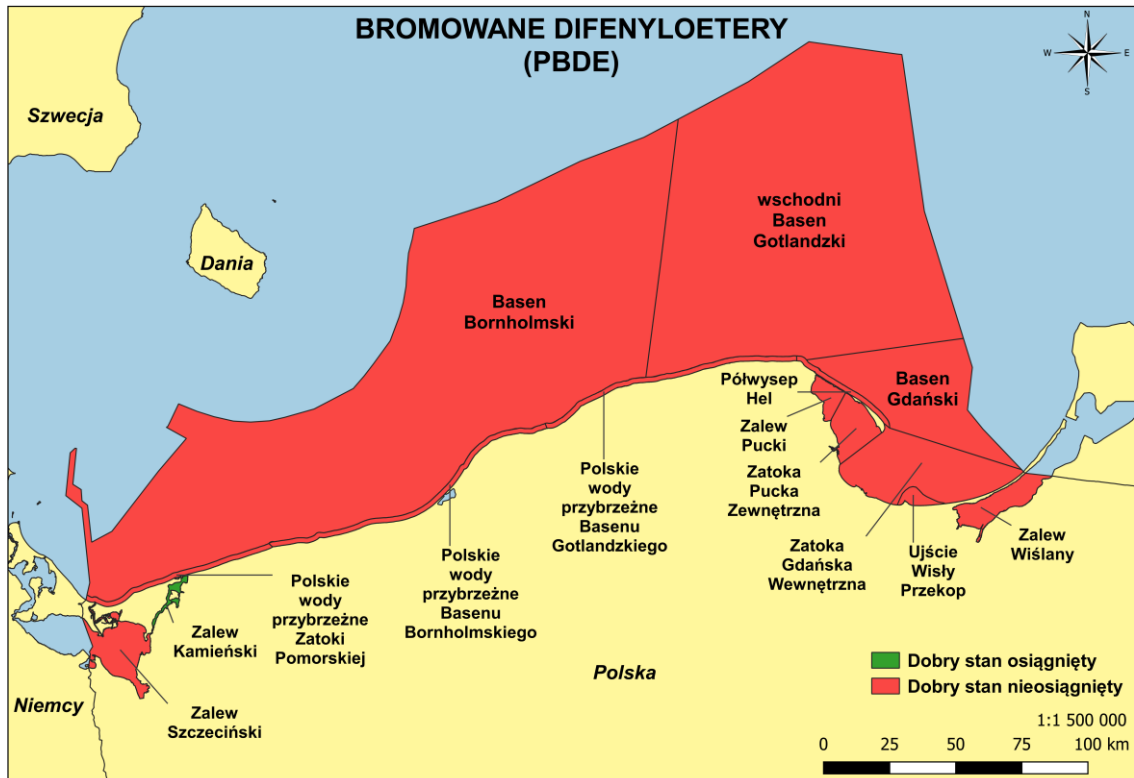
Rysunek 1. Ocena stanu środowiska obszarów morskich w zakresie wskaźnika 'Bromowane difenyloetery (PBDE)' – kryterium D8C1
