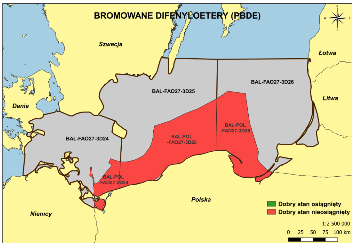
Rysunek 2. Ocena stanu środowiska obszarów morskich w zakresie wskaźnika 'Bromowane difenyloetery (PBDE)' – kryterium D9C1
